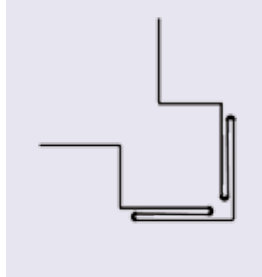
Jambage à cassette, angle extérieur
