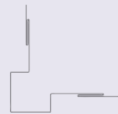
jambage joint debout à cassette, angle sortant
